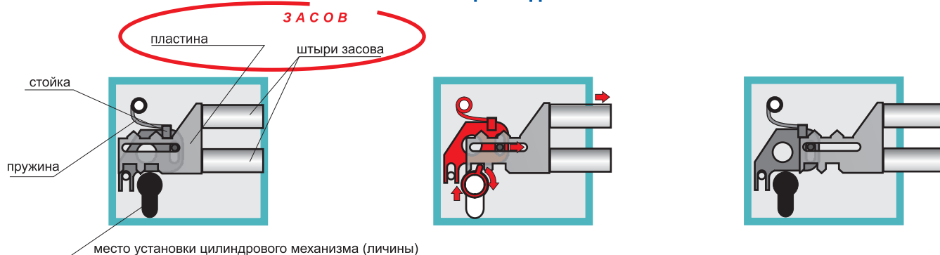
СХЕМА РАБОТЫ ЦИЛИНДРОВОГО ЗАМКА
